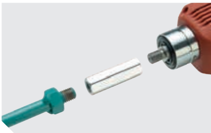
Gewindeanschluss: 49.500-000 1/2" x 20 UNF innen / M 14 innen
