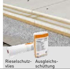
Gebundene Schüttung
