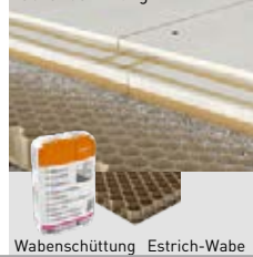
Wabenschüttung Estrich-Wabe
